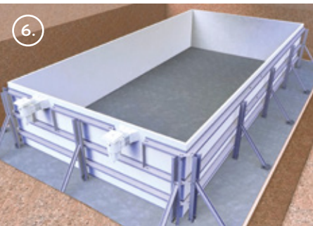
Installer les éléments enterrés (skimmer, refoulement)
