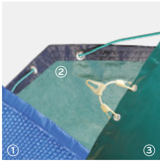
BÂCHES 1. Bâche d'été PE - 400 micron 2. Bâche d'hiver PE - 200g/m² 3. Bâche de sécurité PVC - 580g/m²
